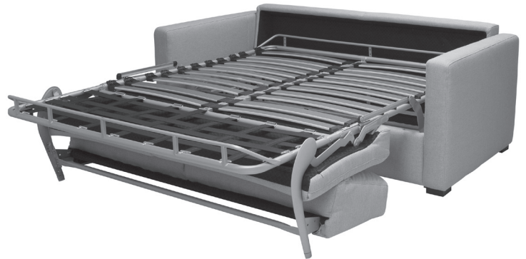
8. Die zweite Armlehne ansetzen. Attach the second armrest.
