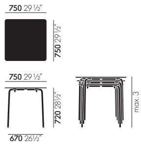
HAL Table, Tischplatte quadratisch
